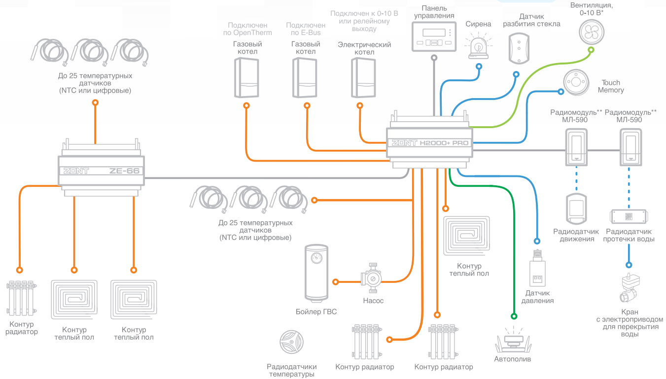
Пример инженерной системы на базе ZONT H2000+ PRO
